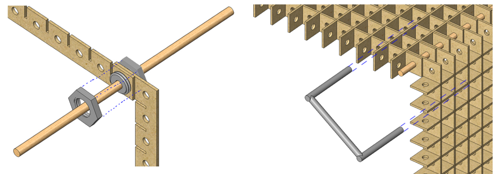
Innesti a pressione bullonati
