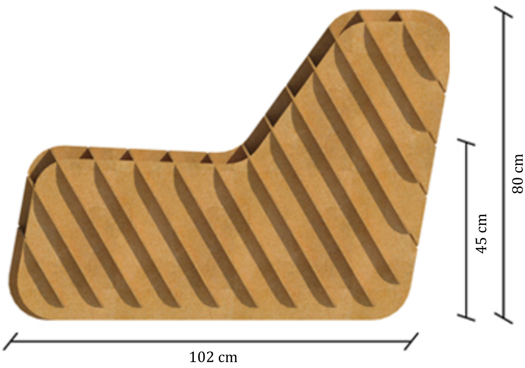
Prospetto laterale
